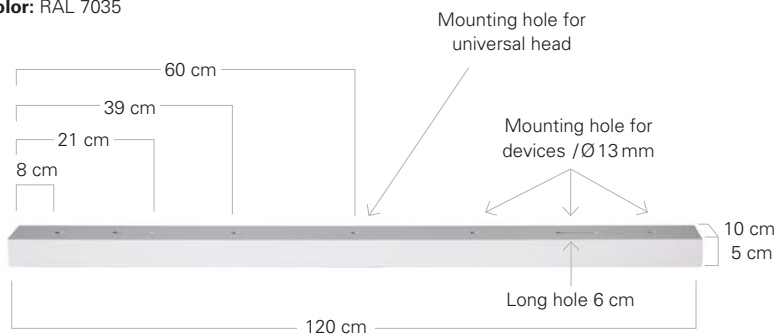
Universal T-Bar
